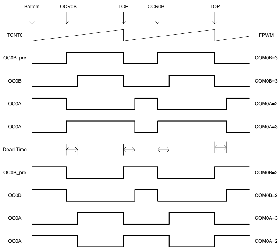
Figure 1 FPWM 模式下 TCO 死区时间控制
