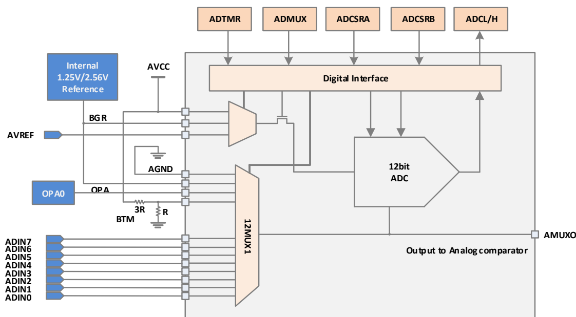
ADC 结构图
