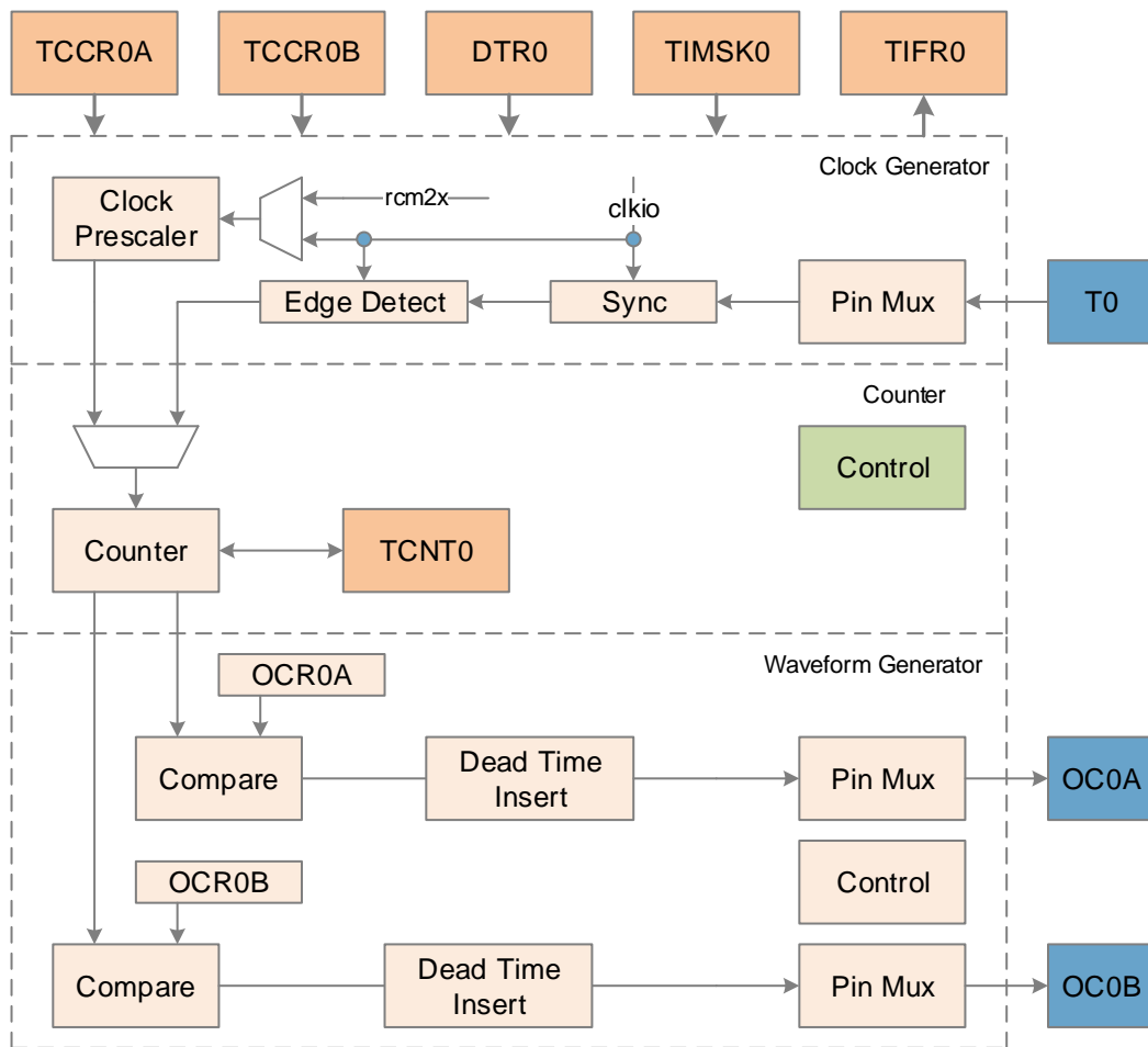
TC0 结构图
