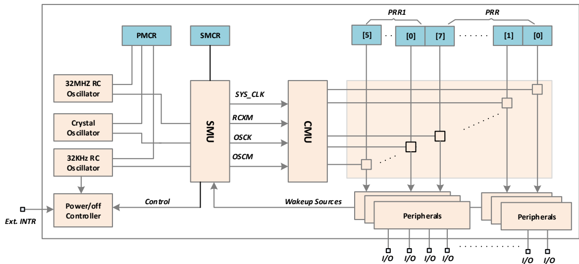
系统功耗管理示意图：
