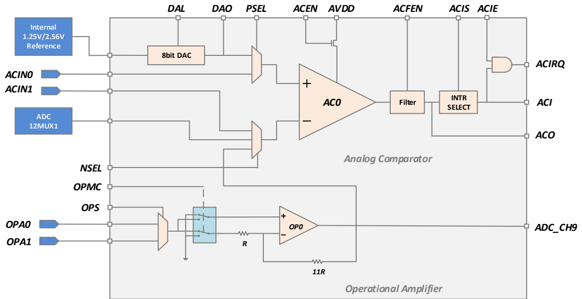
运放/比较器 0 模块结构示意图
