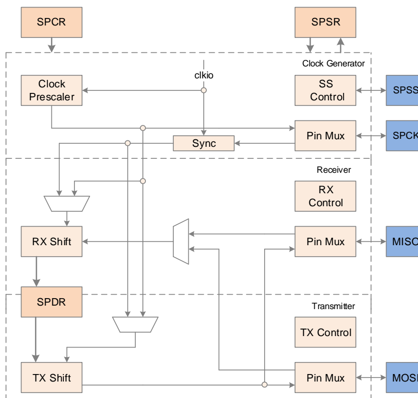
SPI 结构图
