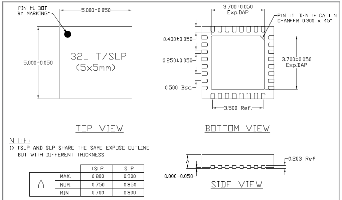
图 6-1. ESP8285 封装
